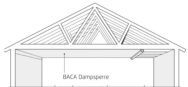
Fig. 2 BACA Dampsperre montert i yttervegg og mot kaldt loftsrom
