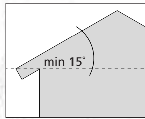
Illustrasjonene viser montering på takvinkel over 15°
