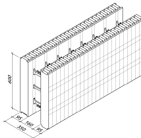
Fig. 1 Vartdal Blokk Standard (mål i mm)
