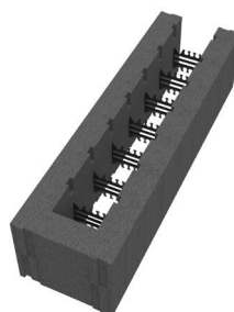
VV23 U-BLOKK TETT H300 X L1200 X B350
