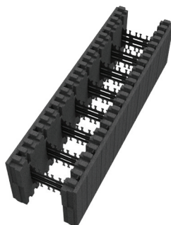
VVD11 BLOKK STANDARD H300 X L1200 X B350
