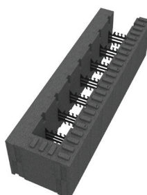
VV29 RADONBLOKK TETT ENDE VENSTRE H300 X L1200 X B350
