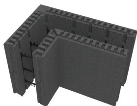
VV02 BLOKK 90° HJØRNE H600 X L900 / 600 X B350
