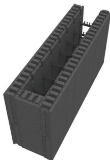
VV03 BLOKK TETT ENDE H600 X L1200 X B350
