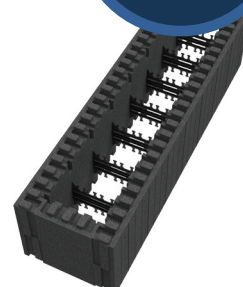
VVD13 BLOKK TETT H300 X L1200 X B350
