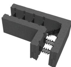
VV22 U-BLOKK 90° HJØRNE H300 X L900 / 600 X B350
