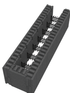
VV13 BLOKK TETT ENDE H300 X L1200 X B350
