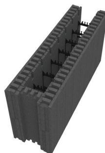
VV04 BLOKK TETT MED UTSP. H600 X L1200 X B350
