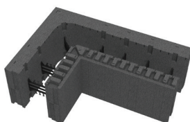
VV28 RADONBLOKK 90° HJØRNE INNVENDIG H300 X L900 / 600 X B350
