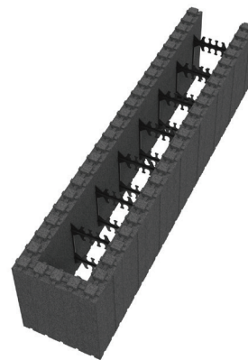
VV25X2 BLOKK TETT H300 X L1200 X B250
