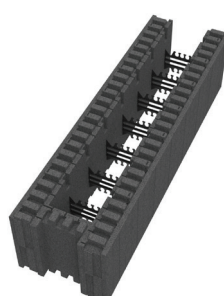
VV14 BLOKK TETT MED UTSP. H300 X L1200 X B350
